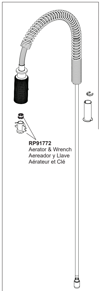
RP103975▲ Spring & Sprayer Assembly Ensamble de resorte y pulverizador Assemblage ressort et pulvérisateur
